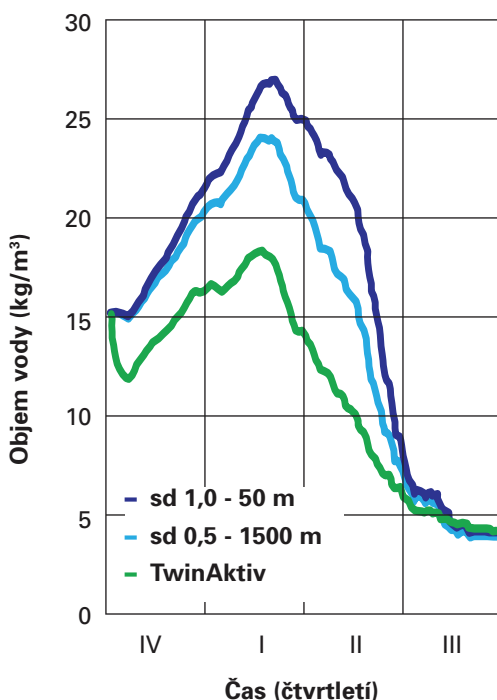
Objem vody v polyuretanové pěně
