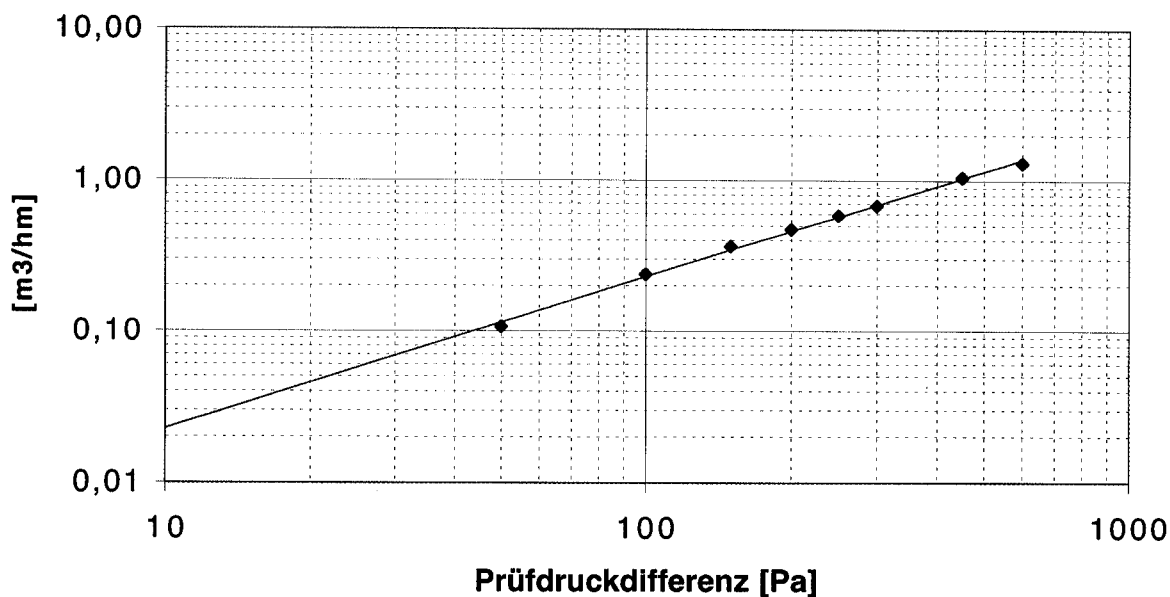
Bild 2: Grafische Darstellung der längenbezogenen Luftdurchlässigkeit (Längsfugen)
