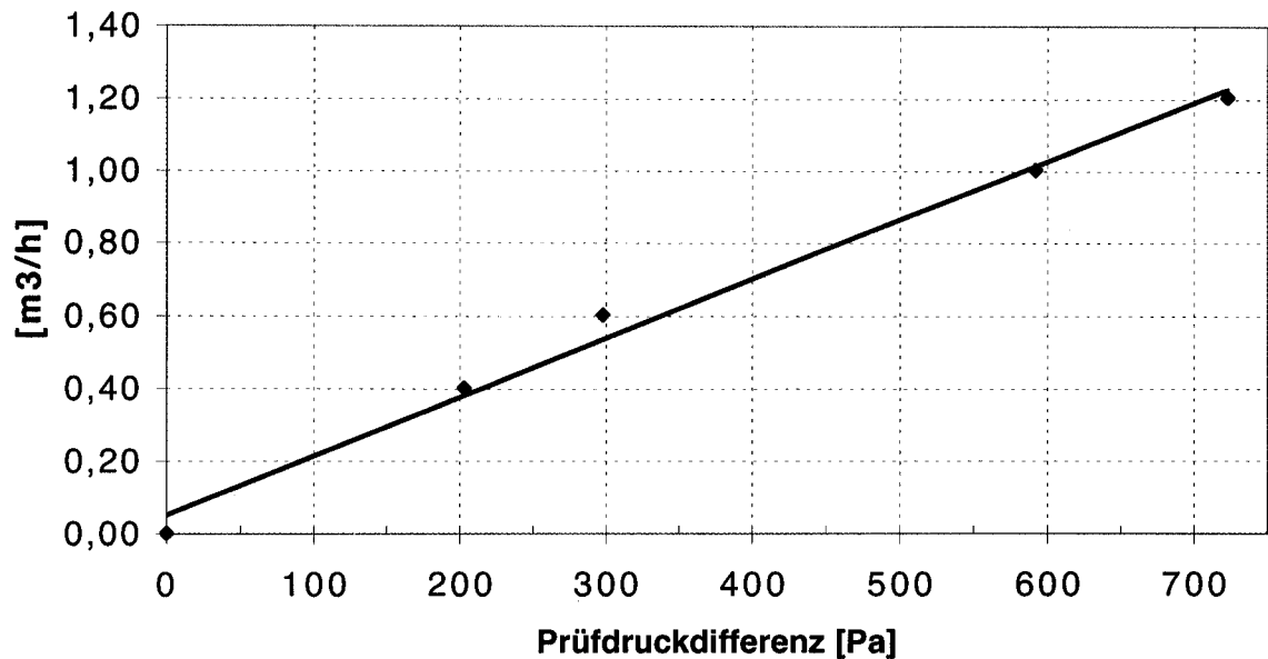
Bild 1: Grafische Darstellung der Prüfstandundichtigkeit (Längsfugen)
